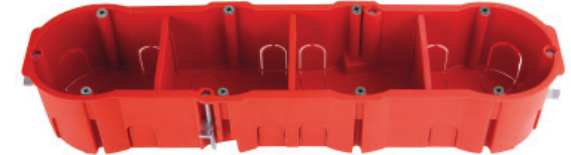
Caja de empotrar 4 elementos para tabique hueco Ref. 2344
